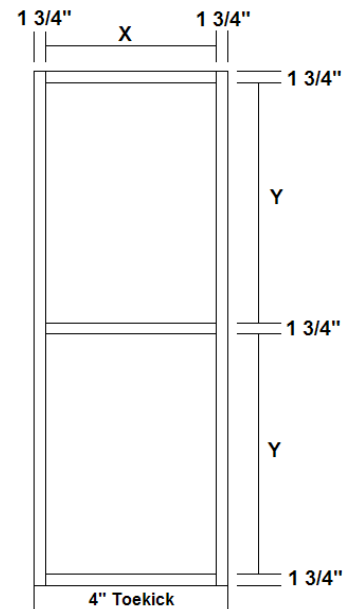
LINEN CLOSET
